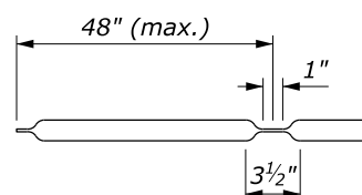
LONGITUDINAL DRAINAGE BAR
