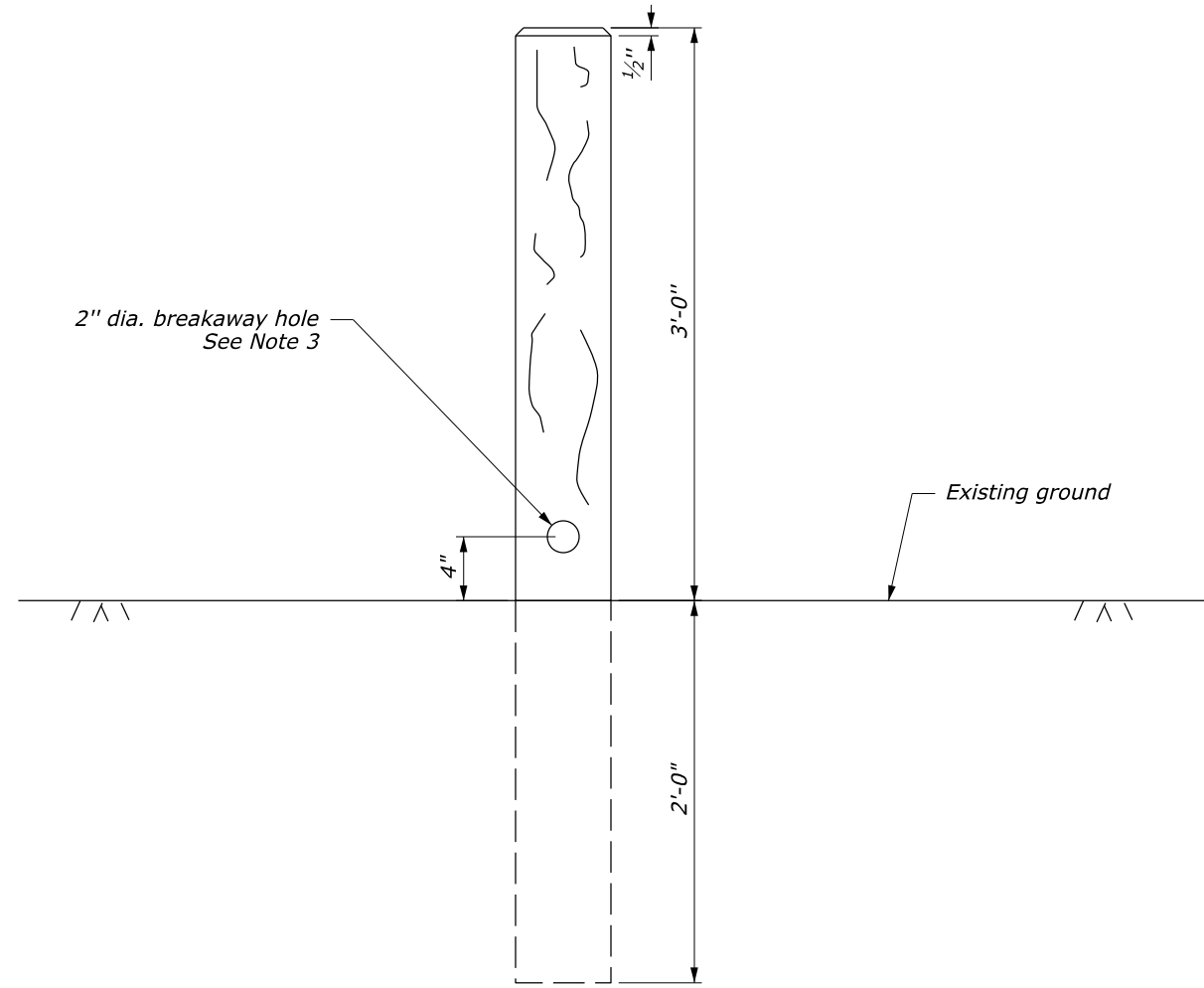
ELEVATION
